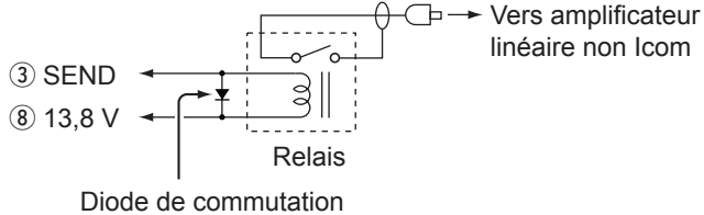
(Exemple) Connecteur ACC
