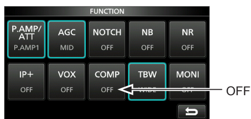
Écran FUNCTION (mode USB)
