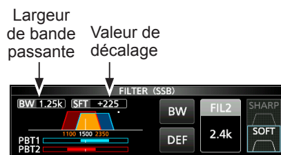
Écran FILTER (SSB) (pendant l'utilisation de Twin-PBT)
